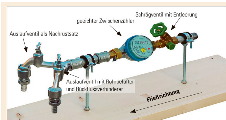
So sollte die Zwischenzählerinstallation aussehen. Das Auslaufventil gibt es sowohl als Komplettsatz als auch als Nachrüstatz. Dieses Modell ist in der Gebührenabteilung des Verbandes ausgestellt.
